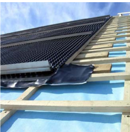
Halterung und Position der Module
