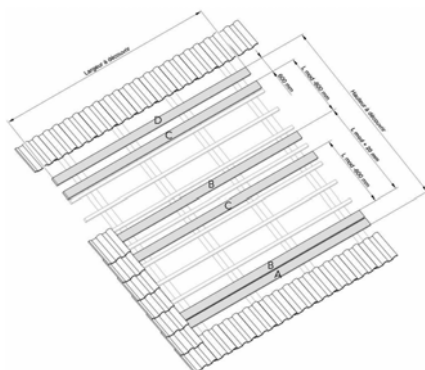
Herstellung des Daches
