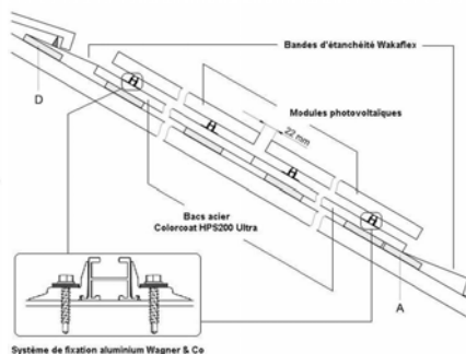
Querschnitt des Befestigungssystems
