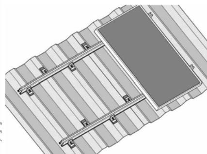
Befestigung der Module auf dem Dach
