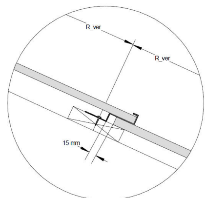
Jonction "Horizontal" entre les laminés solaires
