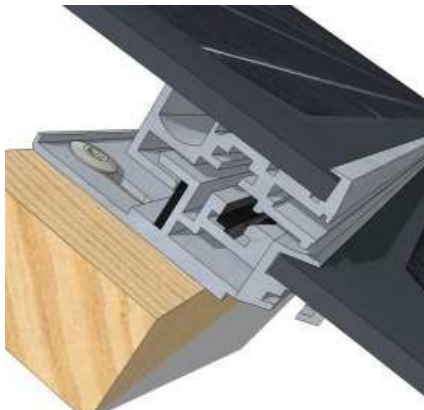
Fixation des modules sur le toit lattes
