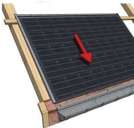
"Bottom line" profil de fixation
