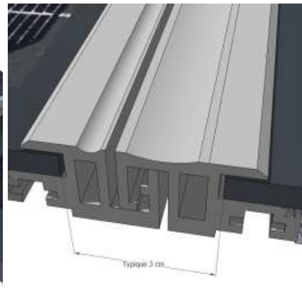
Fixation entre les modules
