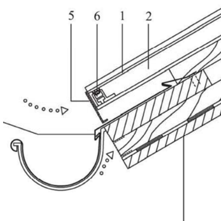
Section gouttière
