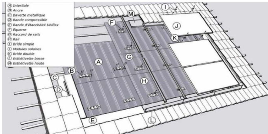
Détails du système de fixation
