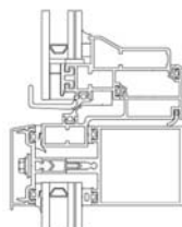
Système et section "Elegance 52 IT"
