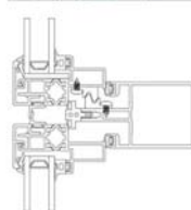
Système et section "Elegance 52 GF"
