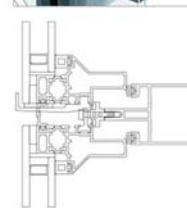
Système et section "Elegance 52 SG TH"
