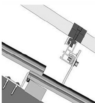
Détail de fixation
