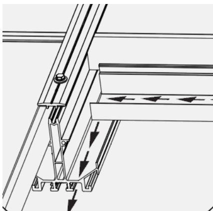
Canaline impermeabilizzanti
