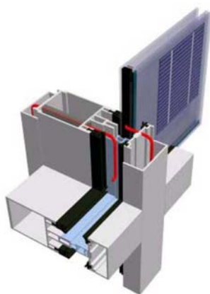
Sezione intelaiatura
