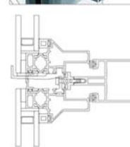
Sistema "Elegance 52 SG TH" e sezione
