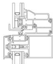
Sistema "Elegance 52 IT" e sezione
