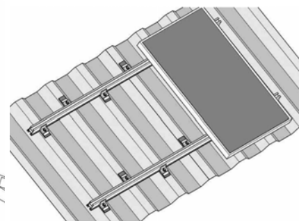
Fissaggio dei moduli sul tetto
