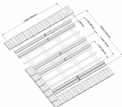
Preparazione del tetto
