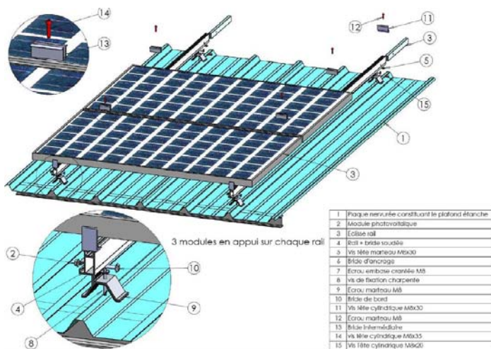
Dettagli del sistema di fissaggio
